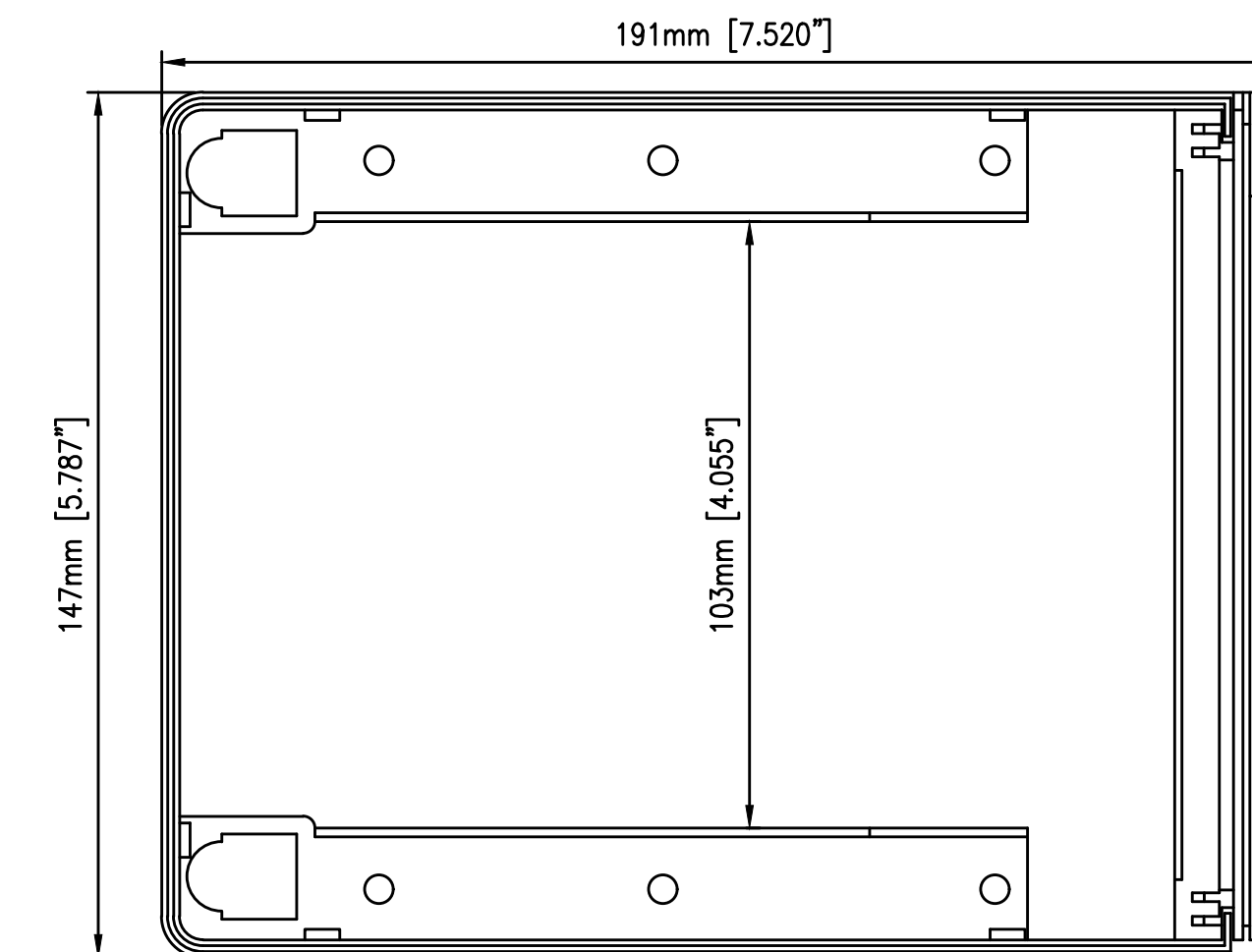
Insert-Bottom
